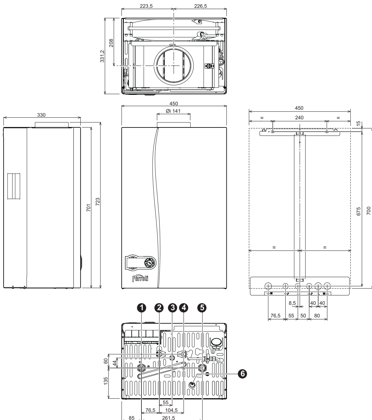
fig. 25 - Dimensioni e attacchi
