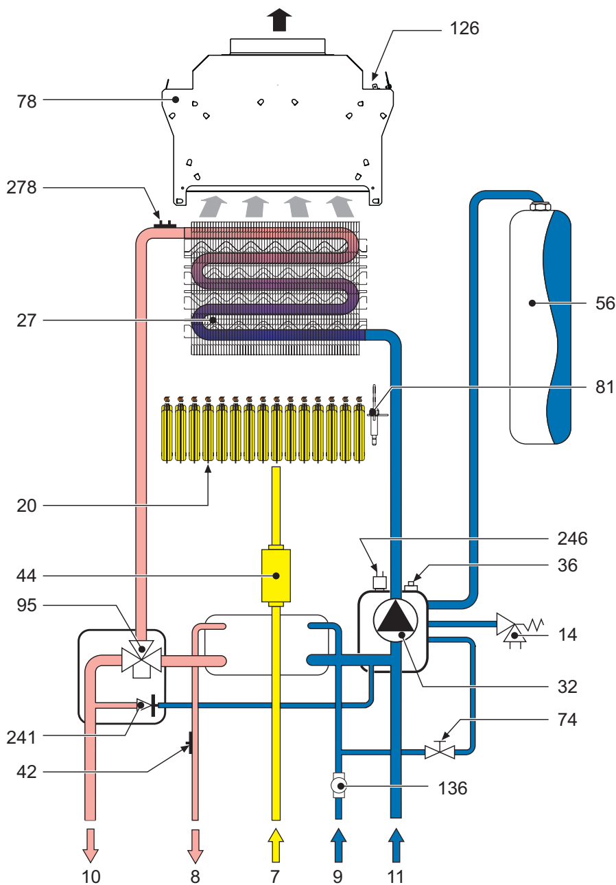
fig. 27 - Circuito idraulico
