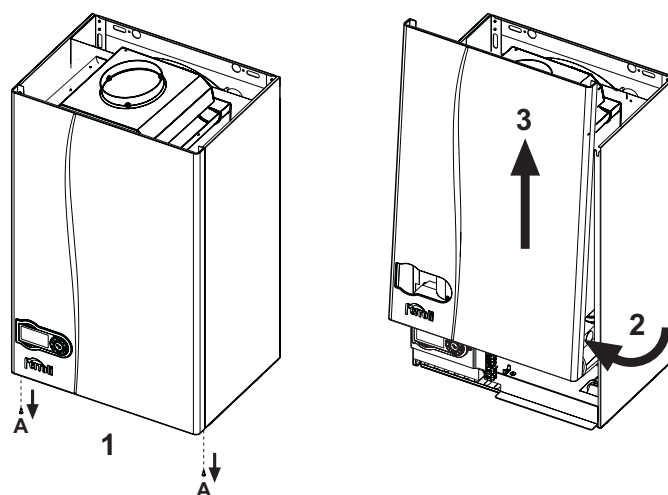
fig. 24 - Apertura mantello
