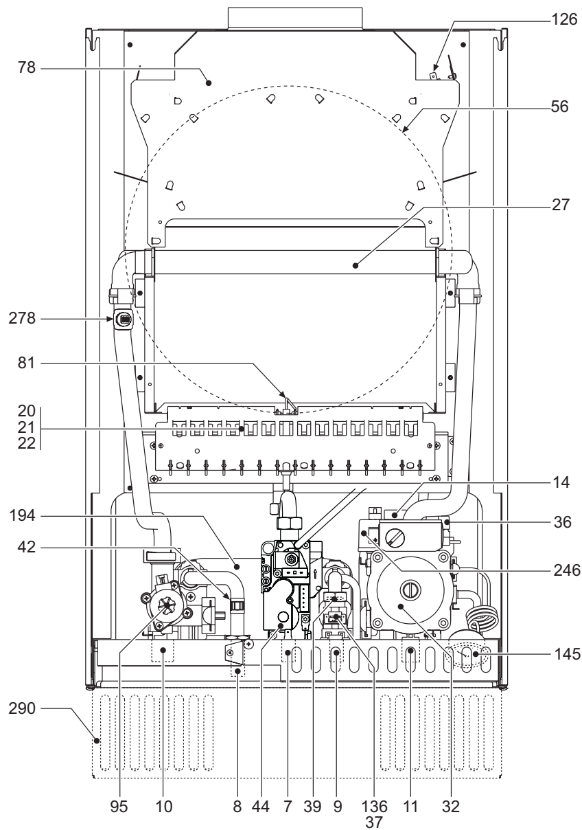
fig. 26 - Vista generale
