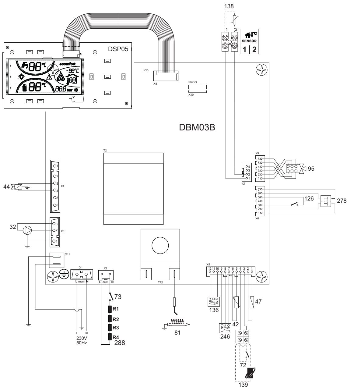
fig. 28 - Schema elettrico
