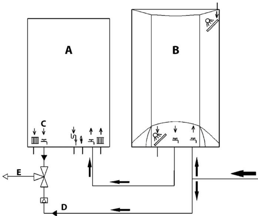
fig. 20 - Schema impianto solare
